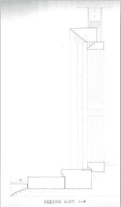
2. Estratto dalla tavola n. 2 del progetto quasi definitivo, sezione A-A
