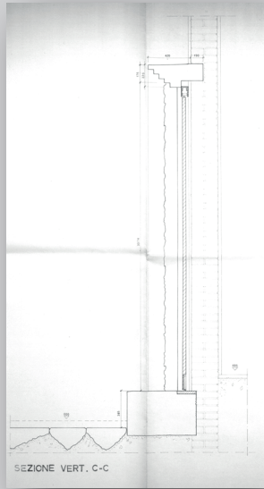
3. Estratto dalla tavola n. 2 del progetto quasi definitivo, sezione C-C
